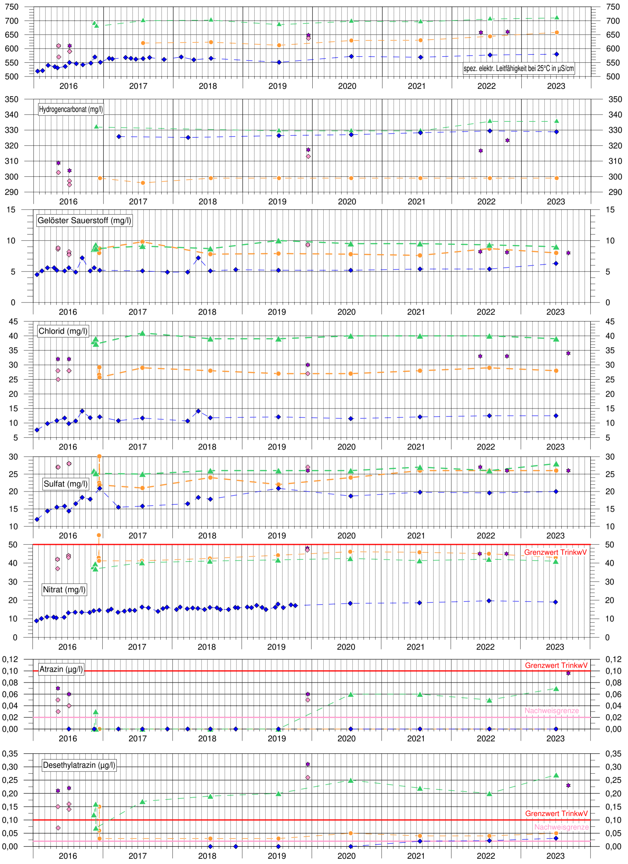
Anlage 14: Darstellung ausgewählter chemisch-technischer Parameter im Wasser aus dem Brunnen I Burghart, den Vorfeldmessstellen GwM 1 Dürnwind und GwM 2 Steig sowie den Grundwassermessstellen Egg T1 und Egg T2 von 2016 bis 2023
