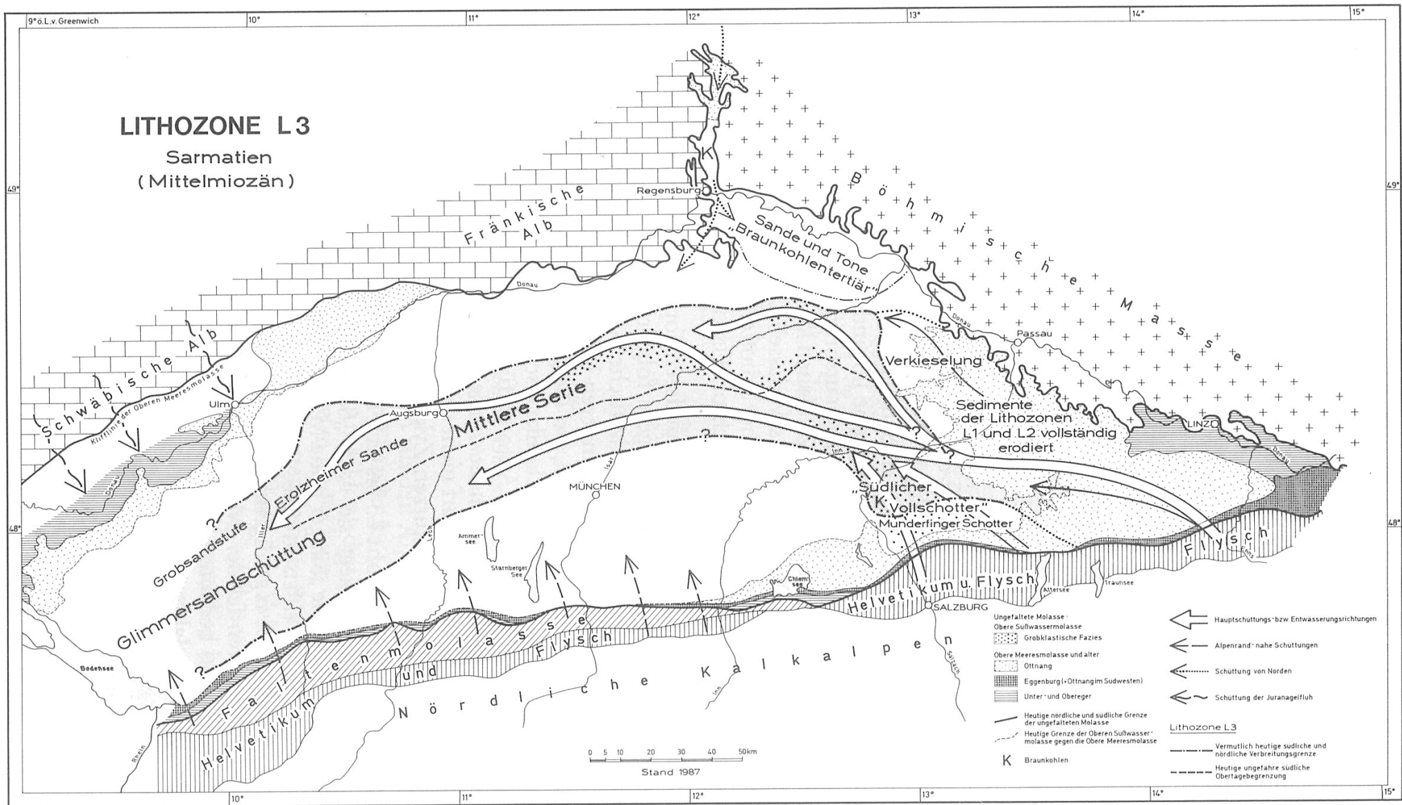
Anlage 2d: Sedimentationsraum der Lithozone L3 (aus UNGER 1989)
