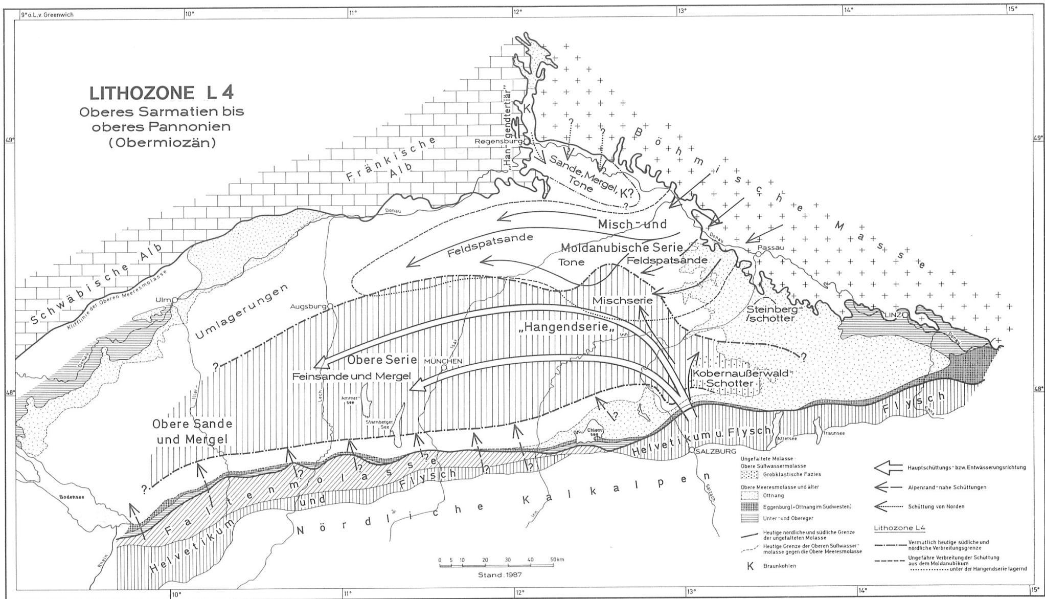
Anlage 2e: Sedimentationsraum der Lithozone L4 (aus UNGER 1989)
