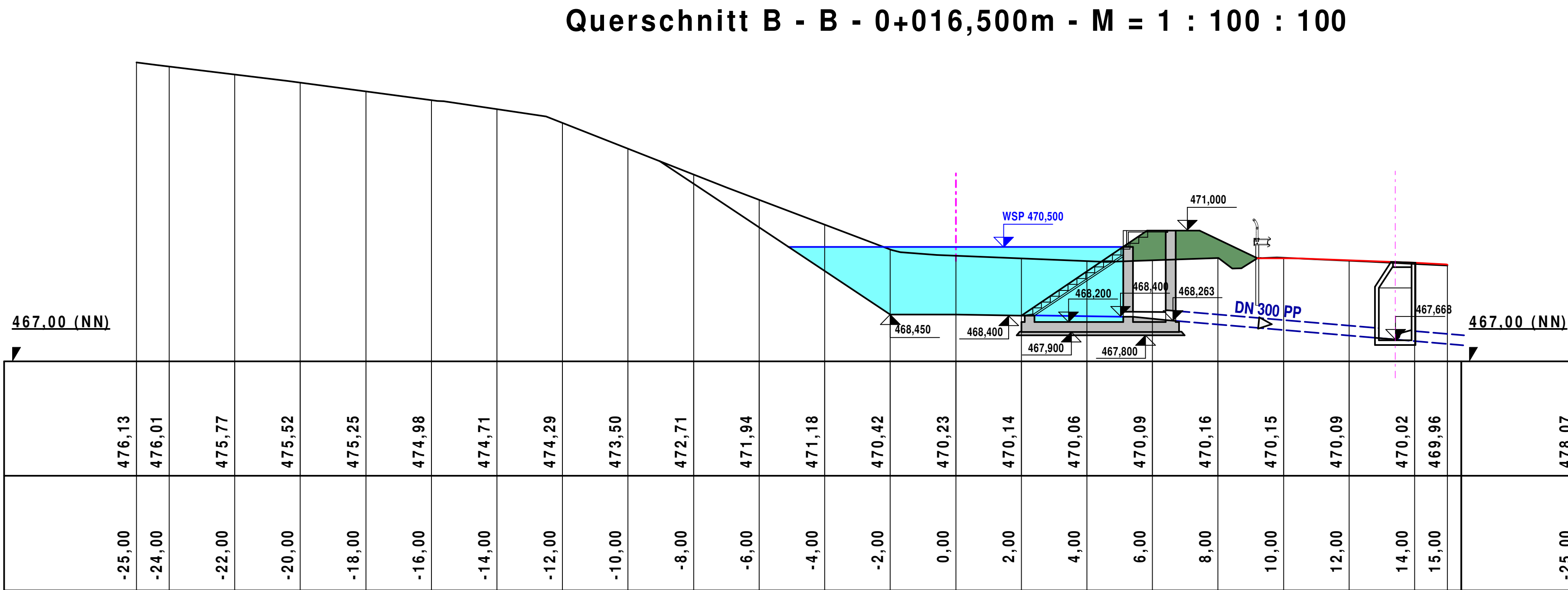
Querschnitt B - B - 0+016,500m - M = 1 : 100 : 100
