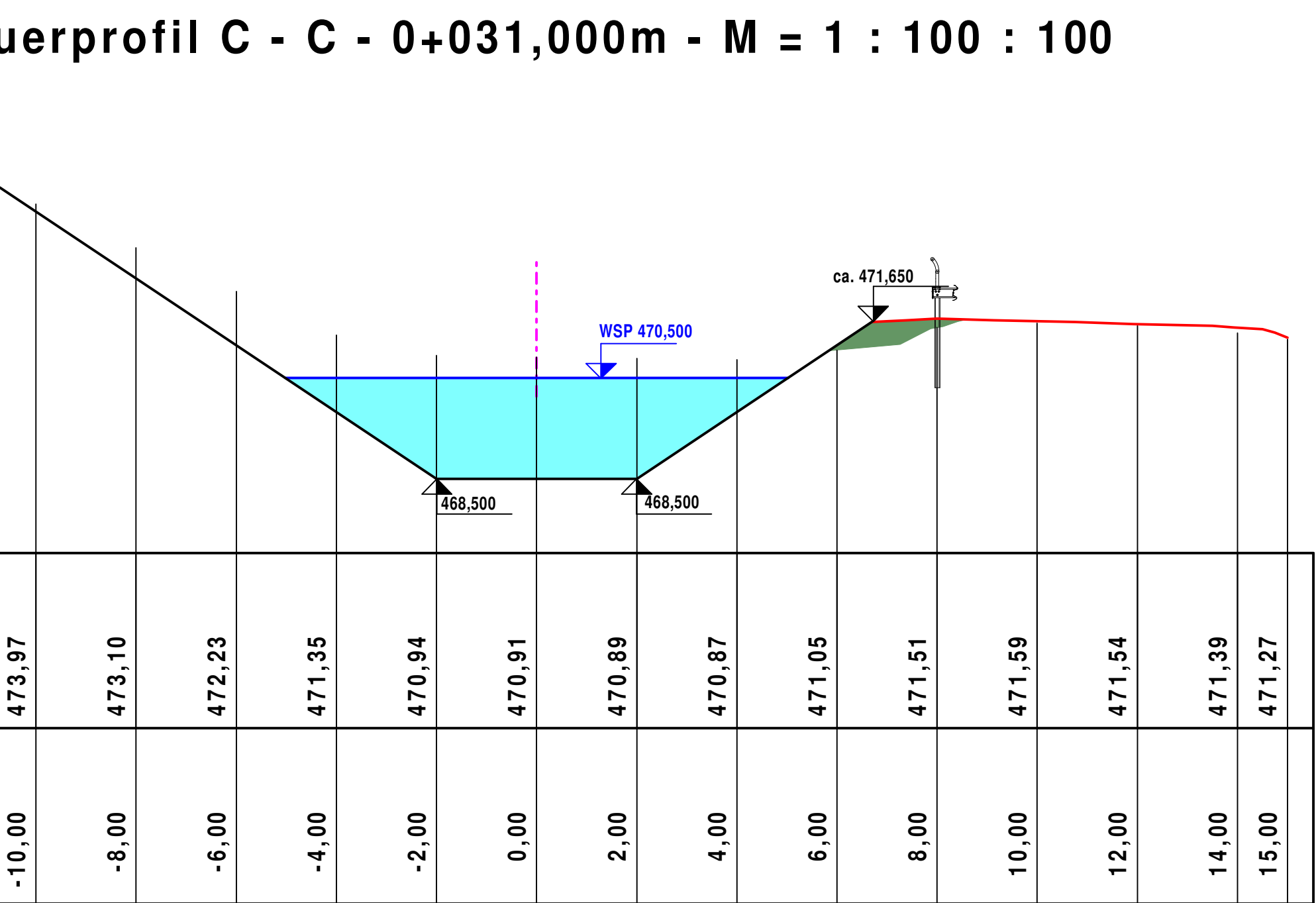
Querprofil C - C - 0+031,000m - M = 1 : 100 : 100
